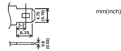
F1 (FASTON TAB NO. 187)
